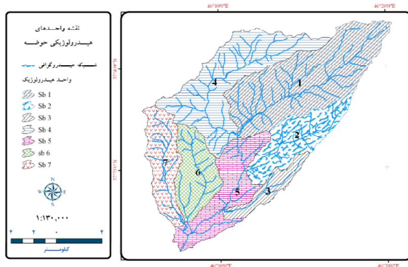
شکل ۴: نقشه‌ی واحدهای هیدرولوژیک حوضه آبریز قلعه‌چای
