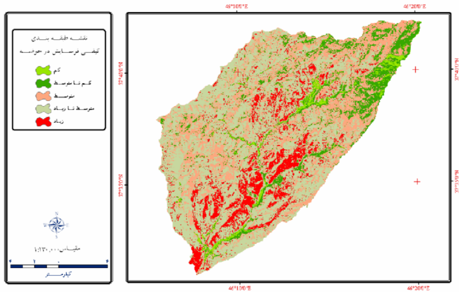
شکل ۹: نقشه‌ی کیفی فرسایش در حوضه‌ی آبریز قله‌چای
