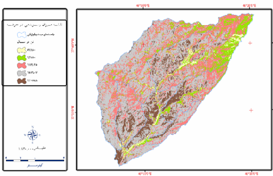
شکل ۱۰: نقشه‌ی میزان رسوبدهی در حوضه‌ی آبریز قله‌چای
