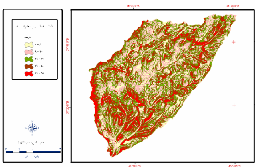
شکل ۶: نقشه‌ی شیب حوضه‌ی آبریز قلعه‌چای
