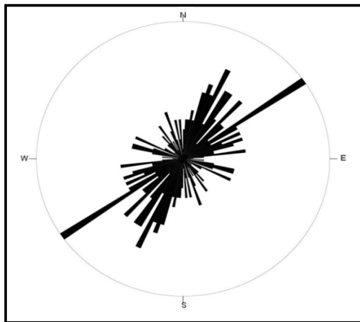
شکل ۶: رزیدیاگرام درزه‌ها در ناودیس ریجاب بر اساس اندازه‌گیری ۲۱۰ درزه با کمپاس مأخذ: نگارندگان
