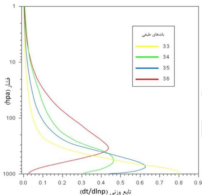
شکل ۱: توابع وزنی باندهای موجود در سنجنده‌ی MODIS واقع در ناحیه جذب \text{CO}_2 برای محاسبه‌ی شفافیت جو (بازسازی شده از کار) Menzel et al., 2010 : مأخذ:
