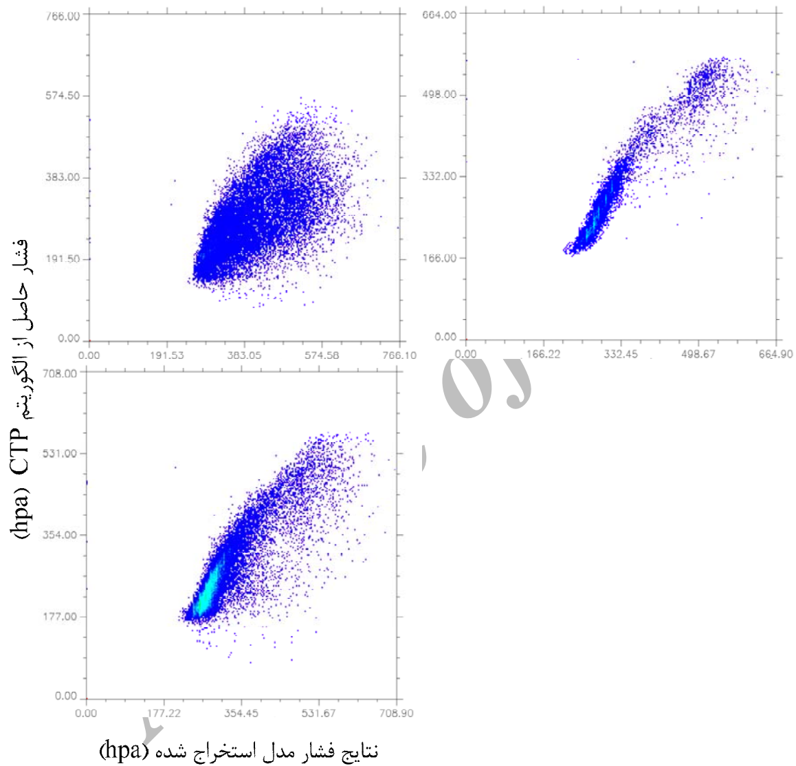
شکل ۱۱: نمودارهای پراکنندگی نتایج حاصل از دو مدل (برحسب هکتوپاسکال)
