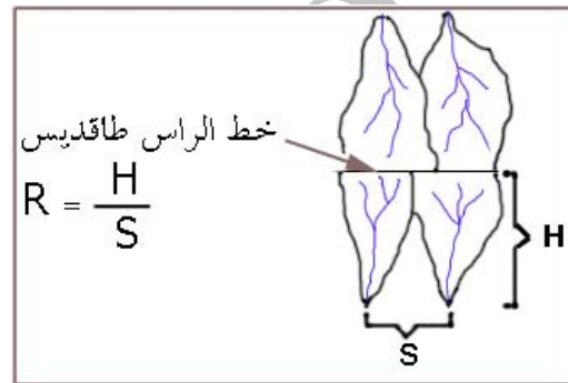
شکل ۸: طرحی شماتیک از نسبت فاصله‌بندی شبکه‌ی زهکشی (R) واقع بر روی پهلوهای طاقدیس
