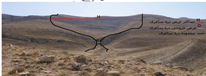
شکل ۵: نمایی از یک دره ساغری در بال جنوبی طاقدیس گلستان
