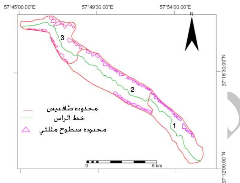
شکل ۷: موقعیت و تعداد سطوح مثلثی شکل در ۳ زون طاق‌دیس گلیان مأخذ: مطالعات میدانی نگارندگان، ۱۳۹۲
