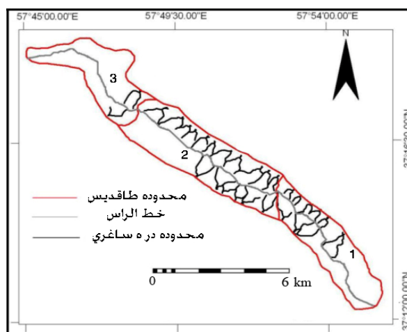
شکل ۴: موقعیت و تعداد دره‌های ساغری در زونهای تکتونیکی طاقدیس گلستان
