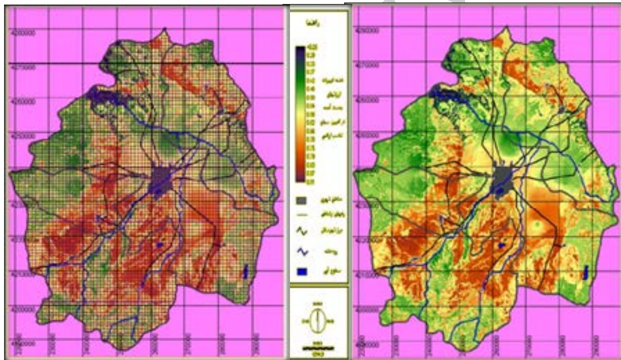
شکل ۴: نقشه سطح بندی شده تناسب اراضی بر مبنای خروجی حاصل از مدل TOPSIS مأخذ: یافته‌های محاسباتی نگارندگان، ۱۳۹۰
