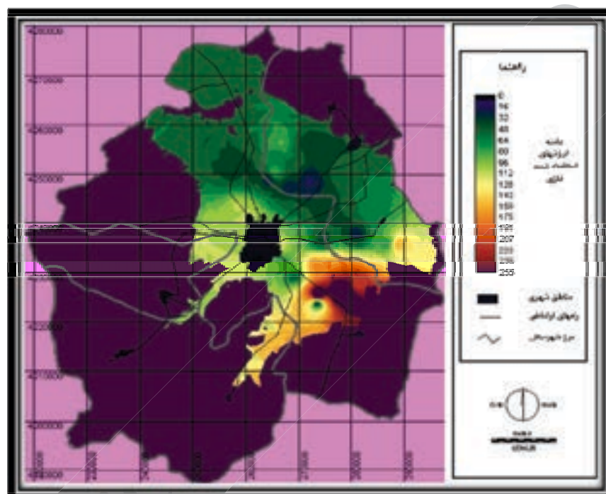
شکل ۲: نقشه ارزش‌های استاندارد شده فازی موقعیت نسبت به سطح آب‌های زیرزمینی مأخذ: بررسی‌ها و محاسبات نگارندگان، ۱۳۹۰
