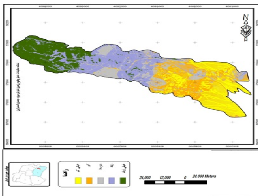
شکل ۶: نقشه طبقات خطر وقوع زمین‌لغزش و پهنه‌بندی درحوزه آبخیز جهان
