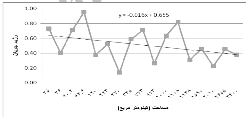
شکل ۱۰: رابطه مساحت و رژیم جریان در دوره‌ی بازگشت ۲ سال
