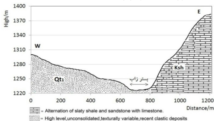
شکل ۱۴: نیمرخ عرضی رودخانه‌ی زاب در فاصله‌ی ۲۵/۳ کیلومتری از دیواره‌ی سد کانی‌سیو (بازه‌ی ج) تهیه و ترسیم: نگارندگان، ۱۳۹۴
