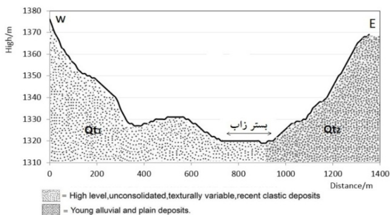
شکل ۱۱: نیمرخ عرضی رودخانه‌ی زاب در فاصله‌ی یک کیلومتری از دیواره‌ی سد کانی‌سیو (بازه‌ی الف) تهیه و ترسیم: نگارندگان، ۱۳۹۴
