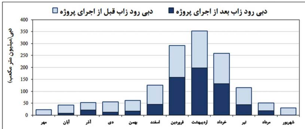
شکل ۶: متوسط دبی رودخانه زاب در ایستگاه گرژال در یک دوره‌ی ۴۹ ساله و دبی آن بعد از اجرای پروژه
