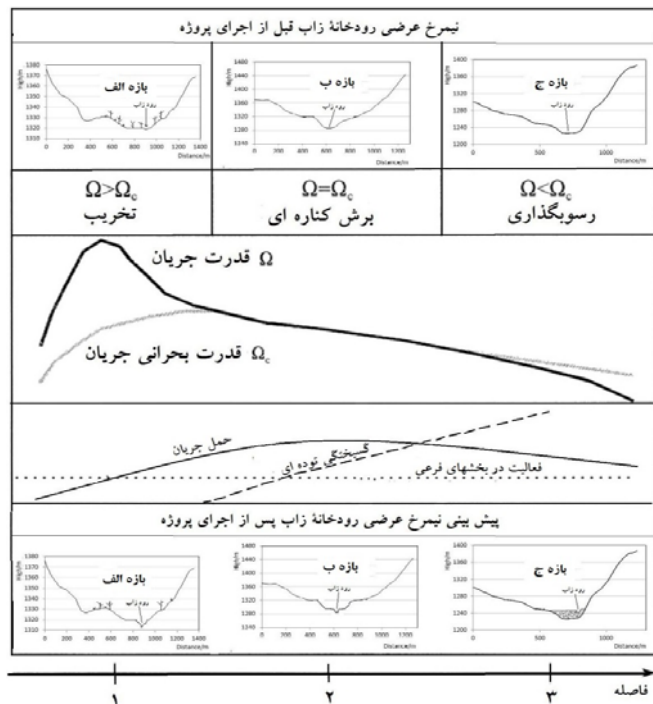
شکل ۱۵: نمایشی از تغییرات قدرت جریان و توان بحرانی رود در پایین دست سد کانی‌سیو و اثرات پروسه‌ی حمل بر فرسایش ترانس‌های کانال تهیه و ترسیم: نگارندگان (Lawler, 1992)
