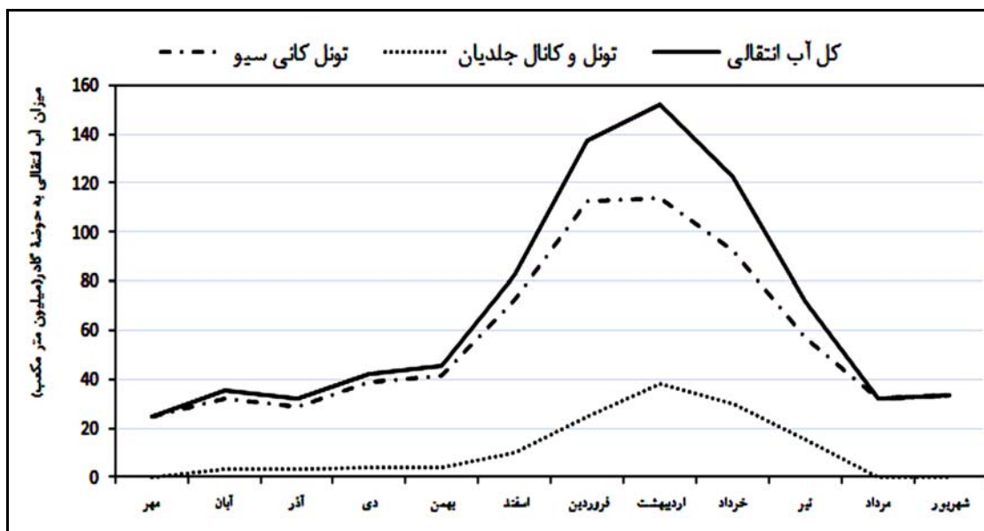
شکل ۳: متوسط بلند مدت میزان بهینه‌ی آب انتقالی از حوضه رودخانه‌ی زاب به حوضه رودخانه‌ی گادار
