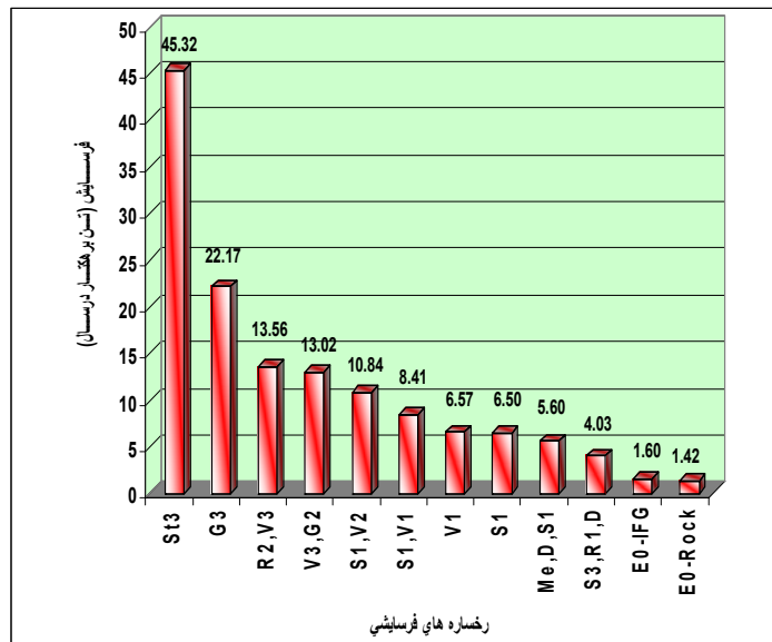
شکل ۱۰: نمودار متوسط شدت فرسایش در هر رخساره فرسایشی
