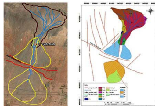
شکل ۱۲: پیدایش مخروط‌افکنه‌های چندبخشی در نتیجه تغییر سطح اساس تهیه و ترسیم: نگارندگان، ۱۳۹۵
