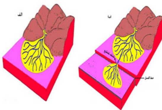
شکل ۱۳: تصویر شماتیک از نحوه ایجاد مخروط‌افکنه‌های چندبخشی تهیه و ترسیم: نگارندگان، ۱۳۹۵
