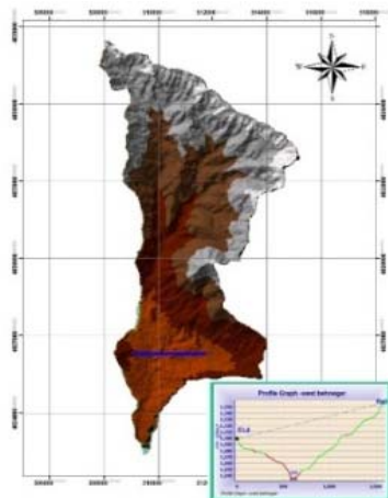
شکل ۲: نحوه‌ی محاسبه پارامترهای شاخص نسبت پهنای کف دره به عمق دره (Vf)
