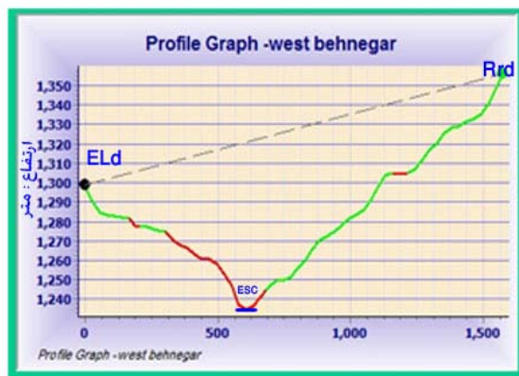
شکل ۲: نحوه‌ی محاسبه پارامترهای شاخص نسبت پهنای کف دره به عمق دره (Vf)
