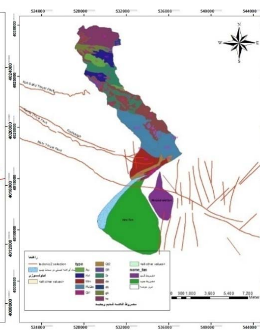
شکل ۱۶: پیدایش مخروط‌افکنه‌های نامتقارن تهیه و ترسیم: نگارندگان، ۱۳۹۵
