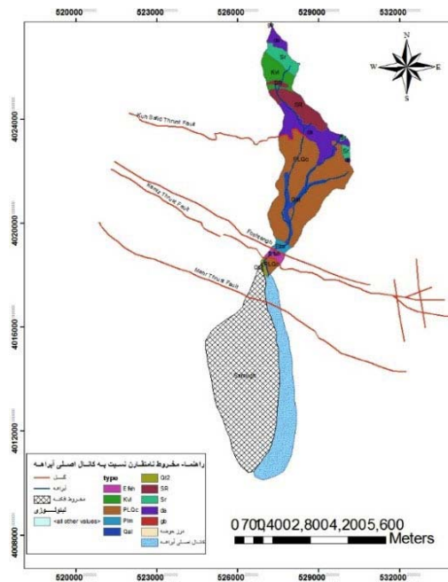
شکل ۱۷: تأثیر تپه‌های مسدود کننده و پیدایش مخروط‌های نامتقارن تهیه و ترسیم: نگارندگان، ۱۳۹۵
