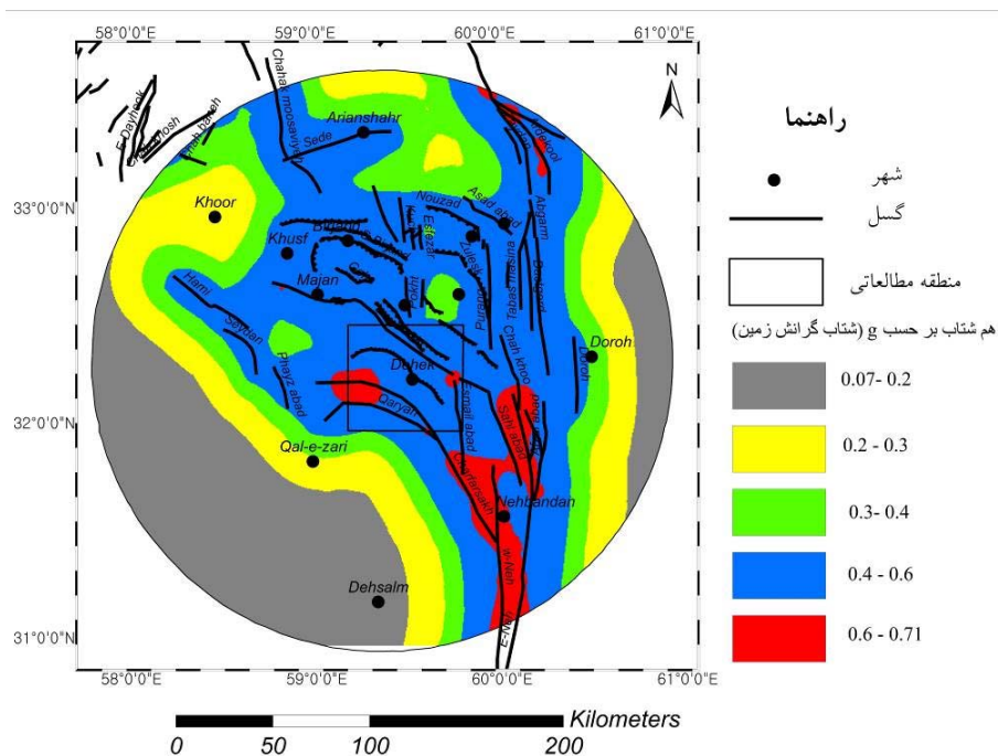
شکل ۳: نقشه هم‌شتاب لرزه‌ای منطقه مورد مطالعه تهیه و ترسیم: محترم قهرمانی، ۱۳۹۵
