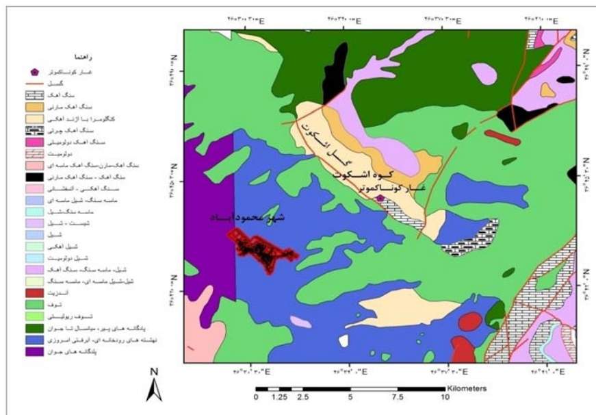
شکل ۲: نقشه زمین‌شناسی کوه اشکوپ مأخذ: نقشه زمین‌شناسی ۱:۰۰۰۰۰ شاهین دژ
