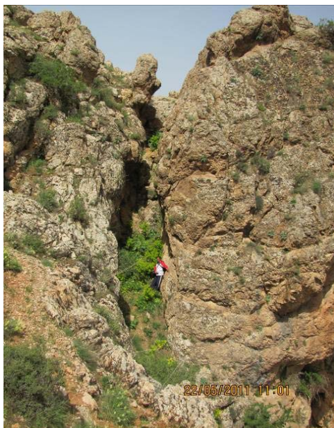
شکل ۳: (سمت راست) نمونه‌ای از یک گریک، شمال غرب کوه اشکوت. (سمت چپ) راهرو انحلالی، دامنه شمالی کوه اشکوت
