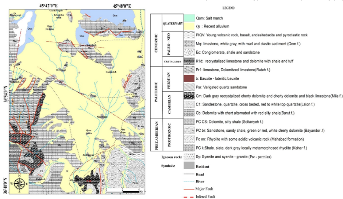
شکل ۲: نقشه زمین‌شناسی محدوده مطالعاتی
