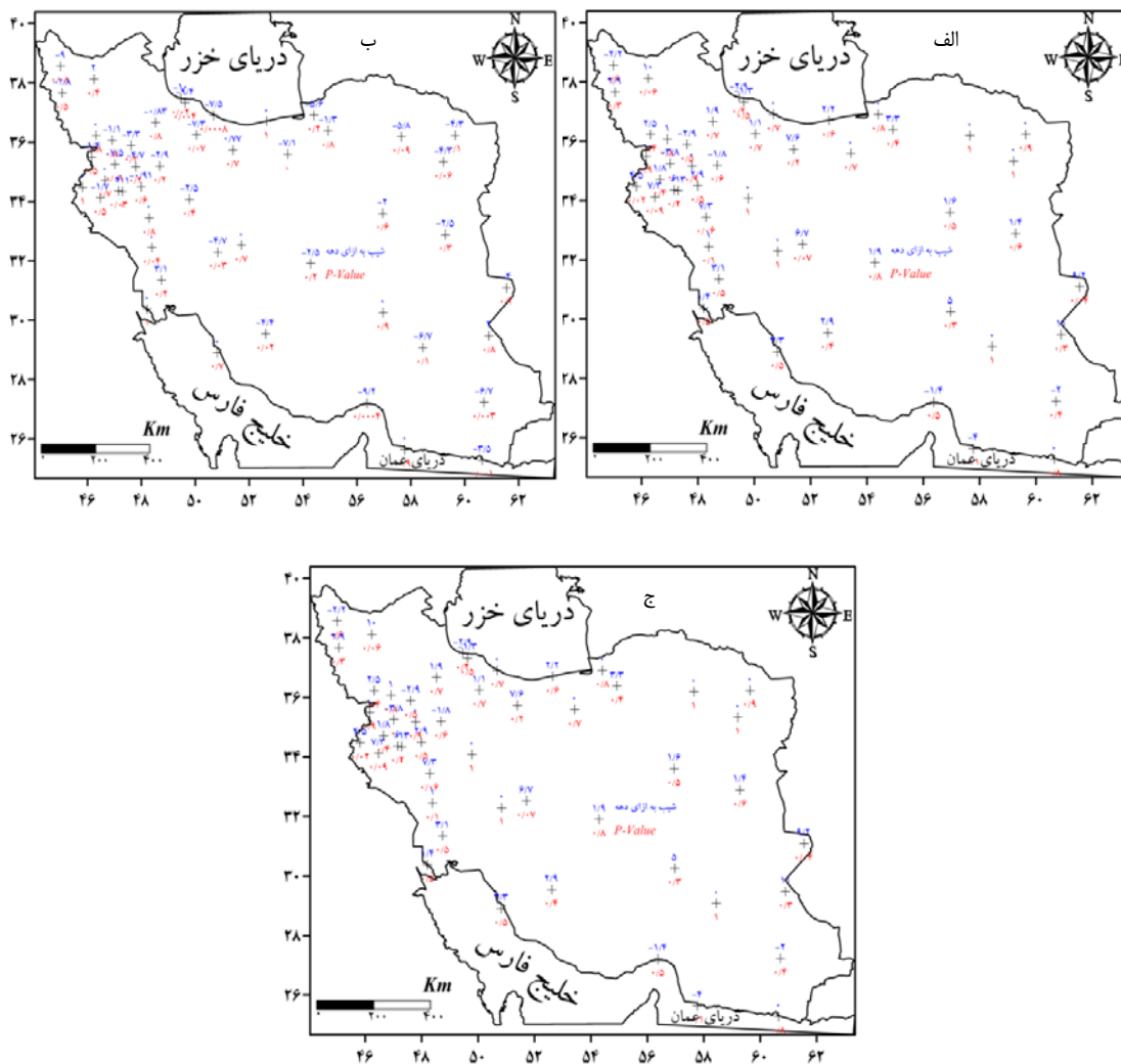
شکل ۶: الف) وردایی آغاز دوره گرما، آهنگ وردایی (آبی) و معناداری (قرمز) آن طی دوره مورد واکاوی بر روی ایران زمین ب) وردایی پایان دوره گرما، آهنگ وردایی (آبی) و معناداری (قرمز) آن طی دوره مورد واکاوی بر روی ایران زمین ج) وردایی طول دوره گرما، آهنگ وردایی (آبی) و معناداری (قرمز) آن طی دوره مورد واکاوی بر روی ایران زمین
