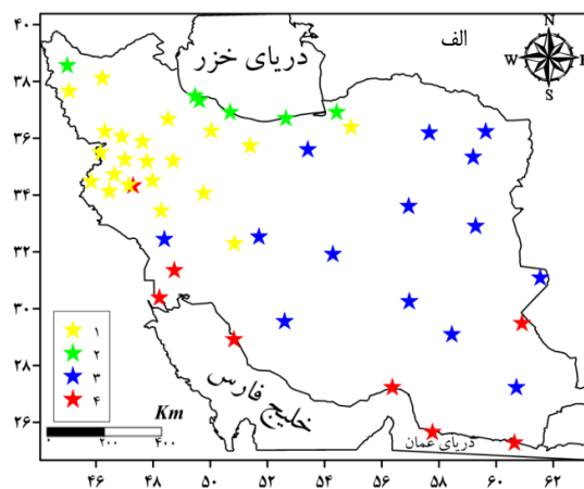
شکل ۵: الف) پهنه‌بندی ایستگاه‌ها براساس طول دوره گرم؛ ب) دارنمای پهنه‌بندی ایستگاه‌ها براساس طول دوره گرم
