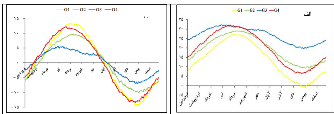
شکل ۳: الف) آهنگ میانگین بلندمدت دمای چهار ناحیه شناخته شده در طول سال ب) آهنگ میانگین بلندمدت انحراف معیار دمای چهار ناحیه شناخته شده در طول سال تهیه و ترسیم: نگارندگان، ۱۳۹۸
