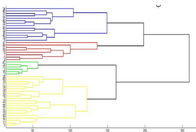
شکل ۵: الف) پهنه‌بندی ایستگاه‌ها براساس طول دوره گرم؛ ب) دارنمای پهنه‌بندی ایستگاه‌ها براساس طول دوره گرم
