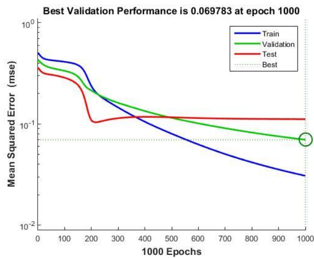
نمودار ۱: منحنی آموزش شبکه عصبی پیشخور
