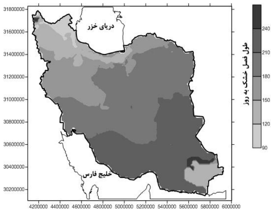
شکل ۴: توزیع مکانی میانگین بلندمدت (۱۹۶۱-۲۰۱۰) طول فصل خشک در ایران
