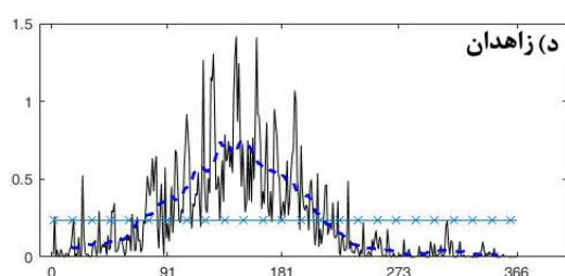
شکل ۲: میانگین مجموع بارش روزانه، میانگین بلندمدت روزانه (۳۶۶ روزه) و میانگین متحرک ۳۰ روزه بارش چهار ایستگاه منتخب تهیه و ترسیم: نگارندگان، ۱۳۹۸
