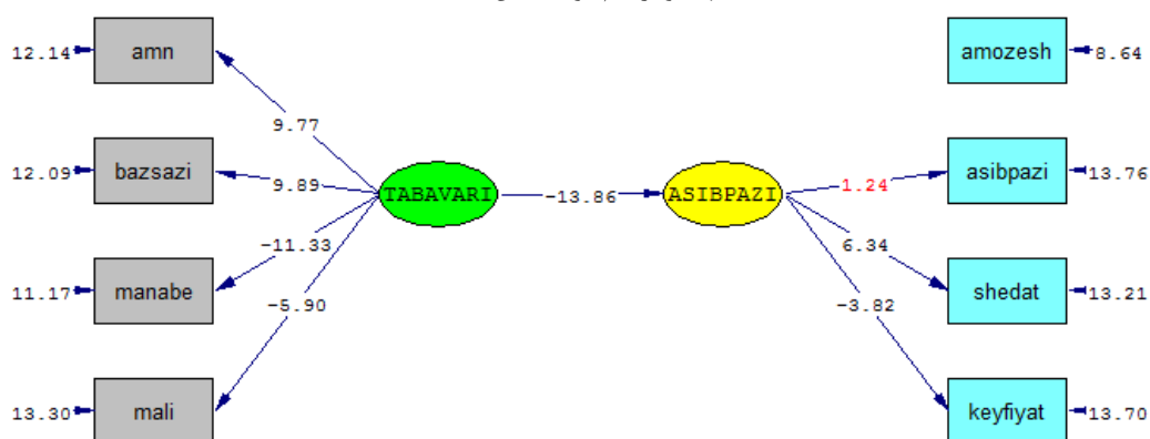
شکل ۴. ضرایب مسیر
