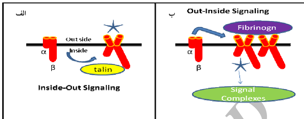
شکل ۱: انتقال پیام دوطرفه در اینتگرین‌ها الف: انتقال پیام از داخل سلول به خارج ب: انتقال پیام از خارج به داخل سلول
