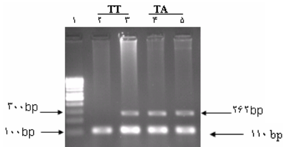
شکل ۱: نمونہ‌ای از نتایج تکثیر ژن IFN-\gamma ستون ۱: 100bp ladder، ستون ۲ و ۴: ویال حاوی پرایمر داری نوکلئوتید T در انتهای ۳، ستون ۳ و ۵: ویال حاوی پرایمر داری نوکلئوتید A در انتهای ۳
