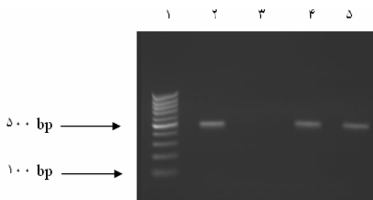
شکل ۲: نتایج تکثیر DNA توسط PCR در اهداءکنندگان خون با HBsAg منفی و anti-HBc مثبت وجود باند ۵۰۰bp نشان دهنده آلودگی به HBV DNA می باشد۔ ladder: ۱: ۲: کنترل مثبت، ۳: کنترل منفی، ۴ و ۵: دو نمونہ مثبت در گروہ مورد و شہادہ
