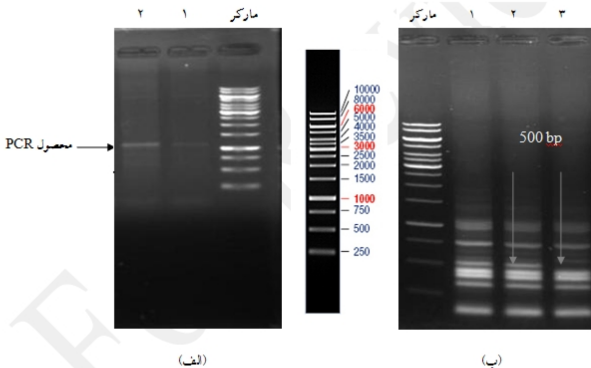
شکل ۴: الف) تصویر الکتروفورز ژل آگاروز یک درصد از PCR انجام شده با پرایمرهای تشخیصی ( A1715 و A1304 ) اریتروپویتین. مارکر DNA ( 1 kb Ladder ). ۱ و ۲: دو سوش انگل ترانسفکت شده با ژن اریتروپویتین. ب) تصویر الکتروفورز ژل آگاروز از PCR انجام شده با پرایمرهای مخصوص اریتروپویتین. مارکر DNA ( 1 kb Ladder ). ۱ و ۲: دو سوش انگل ترانسفکت شده. ۳: انگل ترانسفکت نشده
