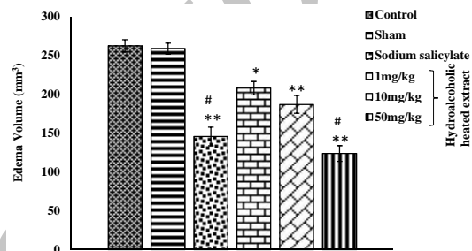
نمودار ۱: مقایسه تغییرات حجم ادم التهابی پا ناشی از تزریق کف پای فرمالین بین گروه‌های کنترل، شم، سالیسیلات سدیم (۳۰۰ mg/kg) و دریافت‌کننده دوزهای ۱ mg/kg، ۱۰ و ۵۰ عصاره هیدروالکلی گل‌های حرارت دیده. نتایج به صورت mean \pm SEM ارائه شده است. * P < 0.01 ، ** P < 0.001 در مقایسه با گروه شم، # P < 0.001 در مقایسه با دوزهای ۱ mg/kg و ۱۰، (n=7)
