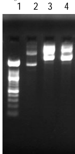
شکل 2- مقایسه پلاسمیدهای استخراج شده بر روی ژل آگاروز 8%/0 نشان می‌دهد که باندهای پلاسمید pT-ROP2 در مقایسه با باندهای پلاسمید pTZ57RT روی ژل آگاروز بالاتر قرار داشتند. ستون 1: نشانگر 100 جفت بازی، ستون 2: پلاسمید pTZ57RT، ستون 3 و 4: پلاسمید حاوی ژن ROP2 (pTROP2).
