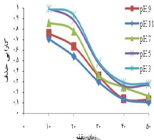
نمودار ۱. اثر pH بر کارایی فرایند الکترو/پرسولفات (دو-کلروفنل ۲۰۰ میلی گرم بر لیتر، ولتاژ ۲۰ ولت، پرسولفات ۰/۰۱ مولار)
