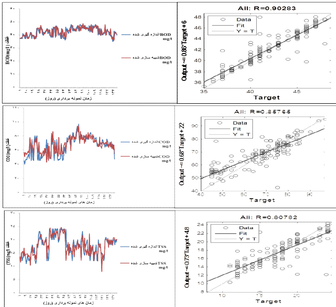
شکل ۱. مقایسه نتایج مقدار BOD، COD، TSS برآورد شده از مدل ANN در مقابل مقادیر اندازه گیری شده
