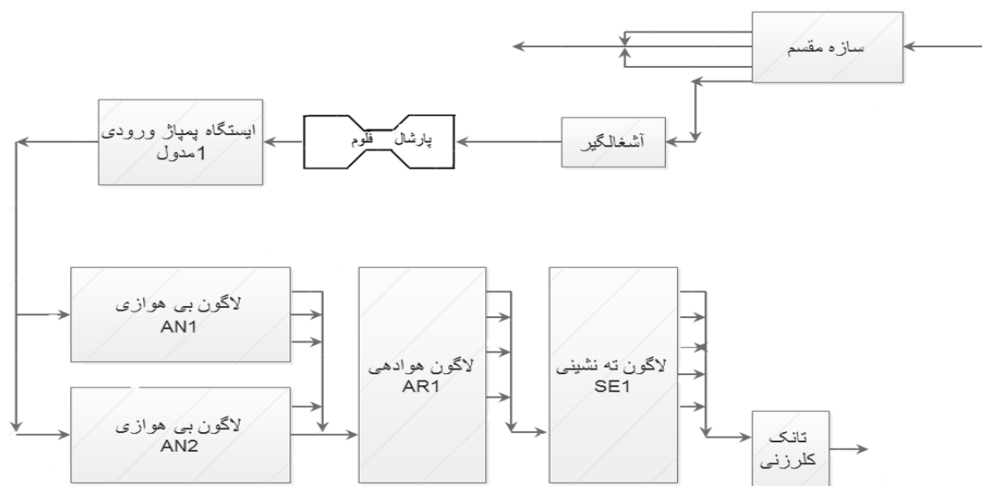
شکل ۱. واحدهای مختلف مدول ۱ تصفیه خانه فاضلاب خرم آباد
