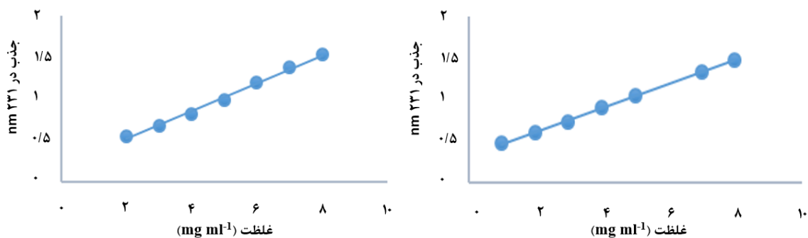
شکل ۱. منحنی استاندارد اسانس اسطوخودوس در حلال ۲-ایزوپروپانول (چپ) و حلال آبی PBS (راست).
