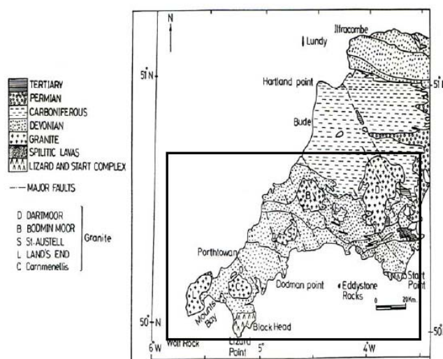
شکل ۳. نقشه زمین‌شناسی ساده شده جنوب غرب انگلستان (کادر مشکی موقعیت برداشت‌های گرانی‌سنجی را نشان می‌دهد).
