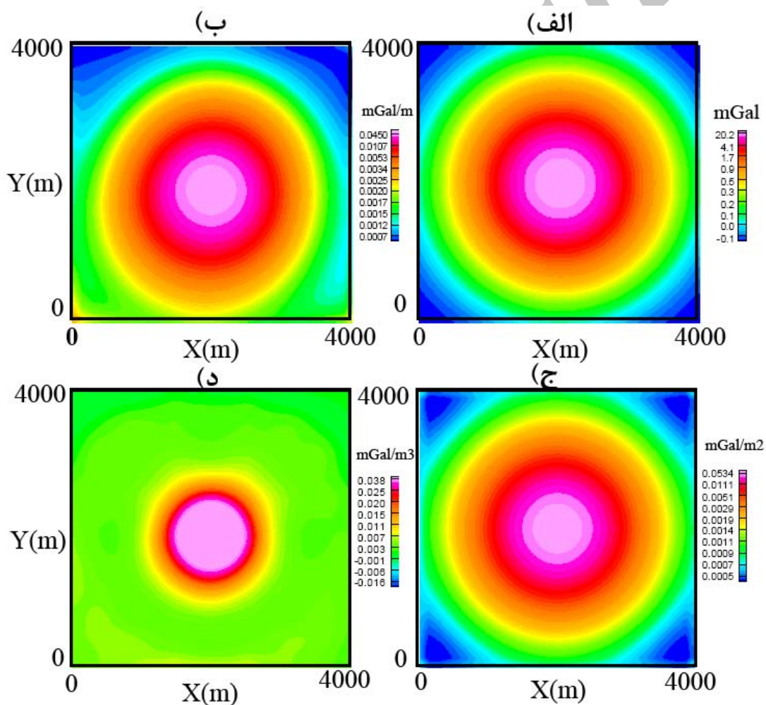
شکل ۲. الف) پاسخ گرانی توده مدل استوانه قائم در عمق ۵۰۰ متری. ابعاد تصویر ۵۰۰×۵۰۰ متر است. ب) نقشه مشتق افقی کل داده‌های گرانی قسمت الف. در این شکل مرزها به صورت متداخل با اطراف برآورد شده است. ج) نقشه سیگنال تحلیلی ساده داده‌های گرانی قسمت الف. د) نقشه مشتق قائم مرتبه دوم سیگنال تحلیلی. در این شکل حدود توده با اطراف با دقت زیادی مشخص شده است.
