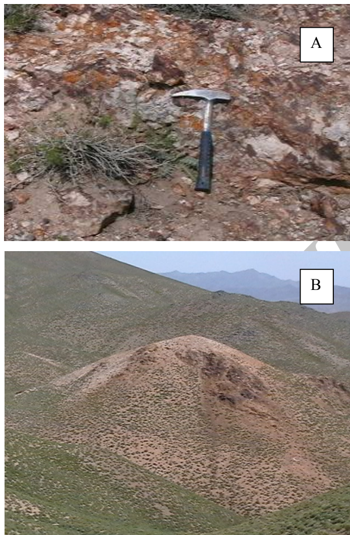
شکل ۱۲. رخنمون‌های مناطق دگرسان شده در منطقه مورد بررسی: A منطقه فیلیک و B منطقه آرژیلیک را نشان می‌دهد. علاوه بر کانی‌های هیدروکسیل‌دار، که به سنگ اصلی رنگ روشن‌تری داده است، اکسید آهن با رنگ قهوه‌ای روی برخی مناطق مشاهده می‌شود.
