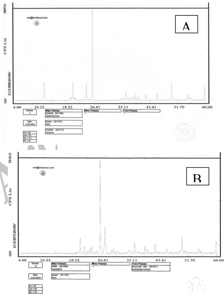
شکل ۱۳. نتایج آنالیز XRD برای ۲ نمونه از دگرسانی‌های منطقه. A- حاوی کانی‌های کائولینیت، کوارتز، و گوتیت و B- حاوی کانی‌های آلپیت، موسکویت، کوارتز و آلپیت.
