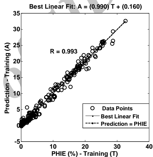
شکل ۱۰. نمودار همبستگی بین تخلخل و برآورد ترکیب آنسامبلی چهارشبکه‌ای شبکه‌های ۱، ۲، ۳ و ۵ به روش خطی بهینه با استفاده از الگوریتم ژنتیک برای الف) الگوهای آموزش و ب) الگوهای آزمون.
