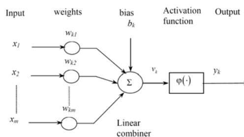
شکل ۱. نمایشی از یک نرون مصنوعی (بات، ۲۰۰۲).
