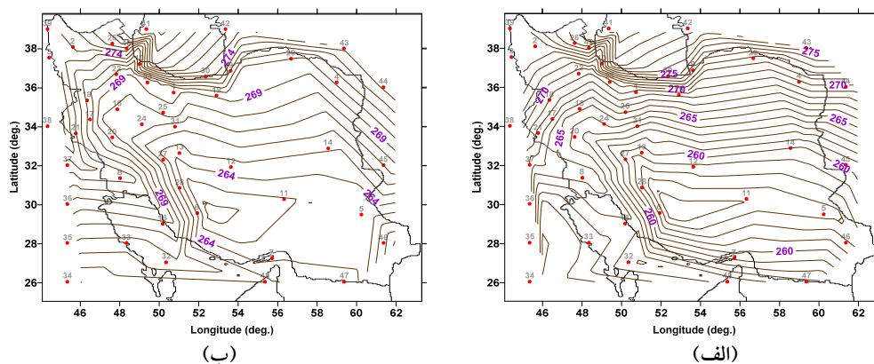
شکل ۱۲. نقشه الگوی پاییزی هم‌مقدارهای ازن کلی در منطقه ایران برای میانگین ماه اکتبر سال‌های (الف) ۲۰۰۷ و (ب) ۲۰۰۸. مقادیر بر حسب واحد دابسون هستند و فاصله هم‌مقدارهای ازن، ۱ واحد دابسون است. نقاط ایستگاه‌ها با شماره مشخص شده‌اند.
