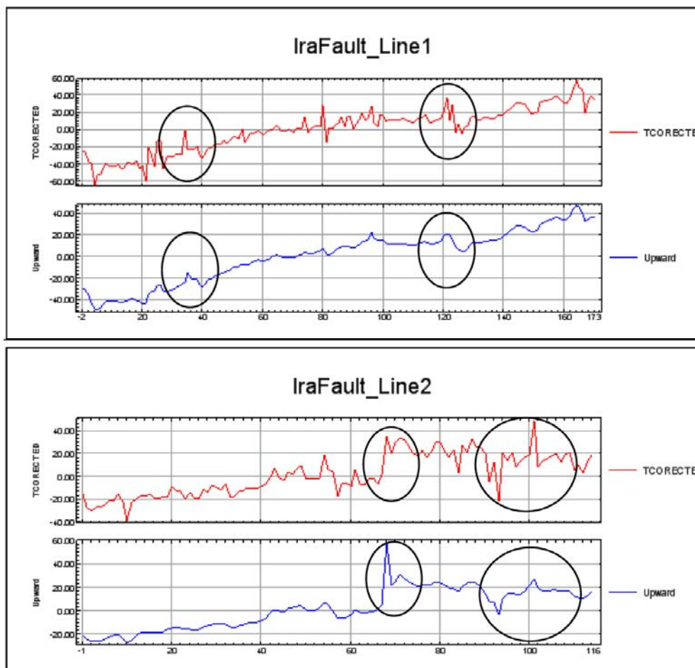
شکل ۳. نمودار داده‌های میدان مغناطیسی پس از اعمال تصحیحات روزانه و IGRF به همراه نمودار ادامه به فراسو تهیه شده برای نیم‌رخ‌های او ۲ با نرم‌افزار Geosoft. در هر شکل نمودار بالایی داده‌های تصحیح شده و نمودار پایینی داده‌های فراسو شده را نشان می‌دهد. ارتفاع فیلتر ادامه به فراسو به صورت تجربی و تا حد حذف نوفه‌های سطحی (بسامدهای زیاد) انتخاب شده است. نواحی محدود به بیضی‌ها، محدوده گسل‌ها را نشان می‌دهند. محور افقی، فاصله به متر می‌باشد.
