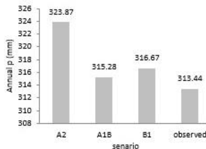
شکل ۹. مقایسه متوسط سالانه بارش شبیه‌سازی شده توسط سناریوهای مختلف و مقدار مشاهده شده در ایستگاه ده بالا
