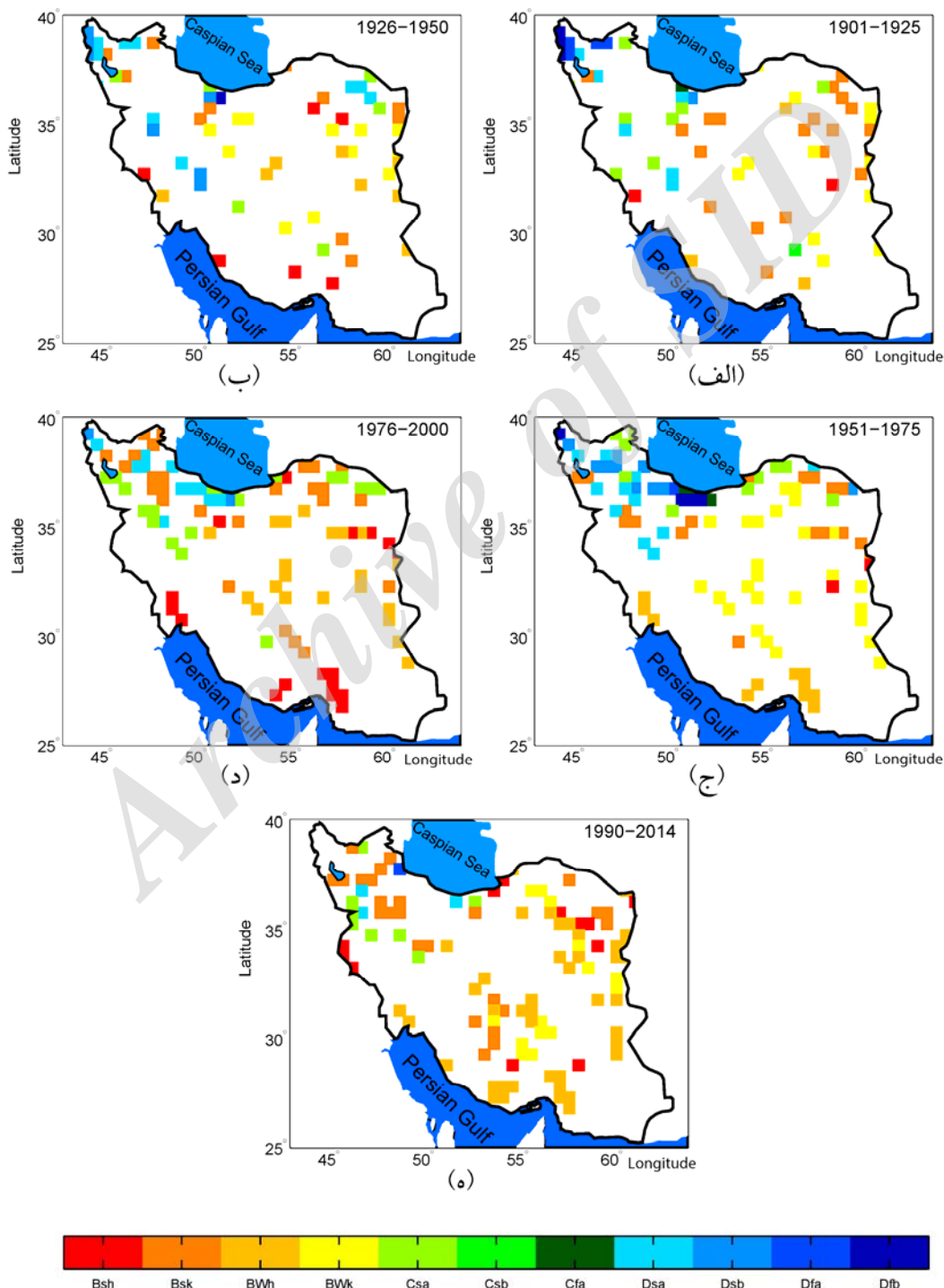
شکل ۹. یاخته‌هایی از گستره ایران که مناطق اقلیمی آن در مقایسه با دوره بیست و پنج ساله آماری پیش‌تر تغییر کرده است.
