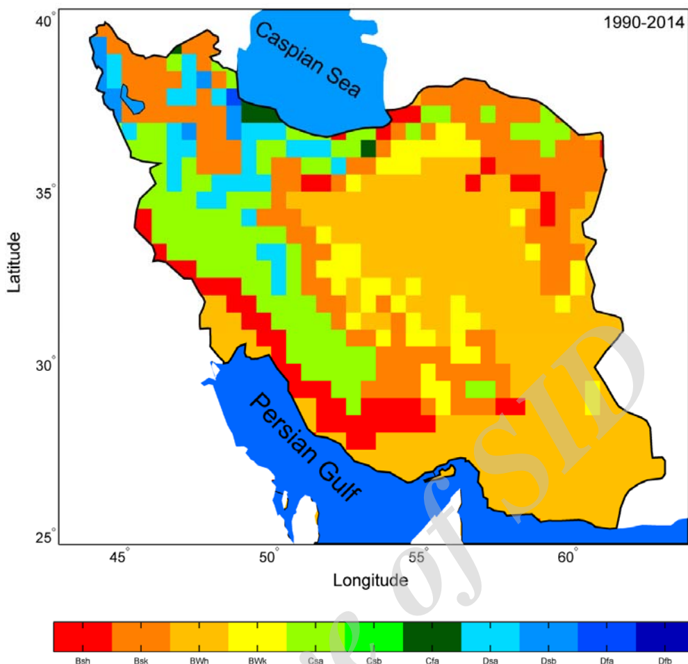
شکل ۷. همانند شکل ۵-ب ولی با استفاده از بارش ماهانه GPCP و میانگین دمای ماهانه CRU در دوره آماری ۱۹۹۰-۲۰۱۴.
