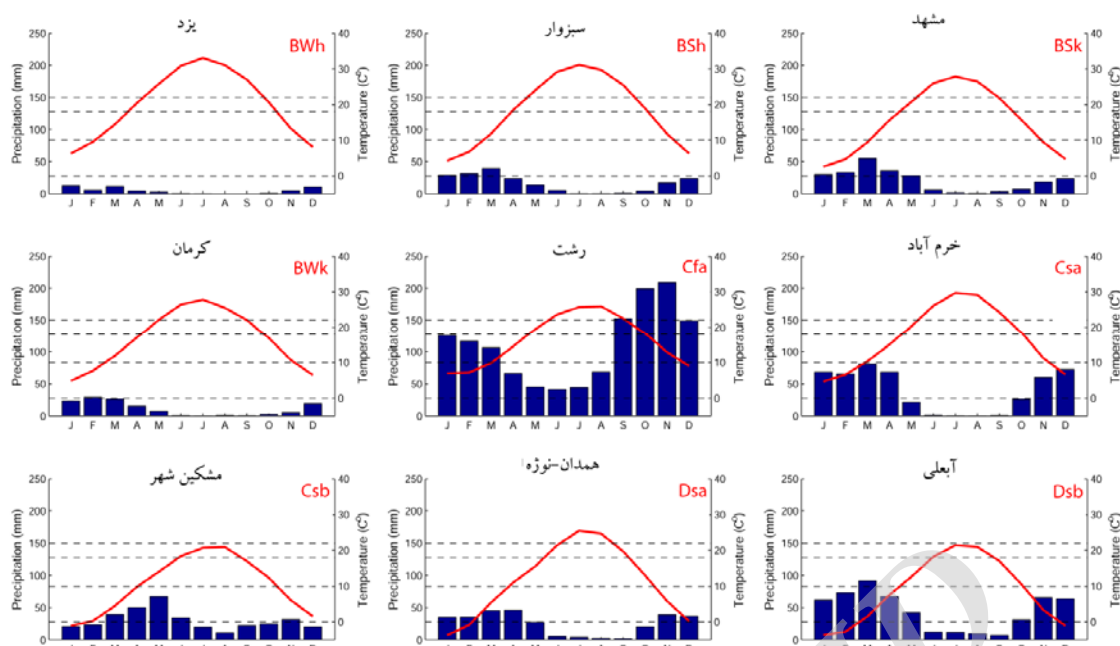
شکل ۶. اقلیم‌نمای کوپن برای ایستگاه‌های معرف گروه‌های اقلیمی موجود در ایران. خط‌چین‌های افقی در برابر دمای صفر، ۱۰، ۱۸ و ۲۲ درجه سانتی‌گراد. آستانه‌های دمایی کوپن-گایگر هستند که به کمک آن نوع اقلیم یک ایستگاه تعیین می‌شود.
