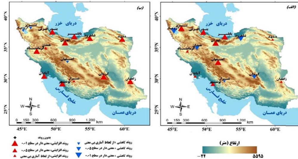
شکل ۶. روند تغییرات متوسط سالانه دمای کمینه در دوره (الف) پیش و (ب) پس از نقطه تغییر؛ نقطه تغییر برای هر یک از ایستگاه‌ها در جدول ۲ نشان داده شده است.
