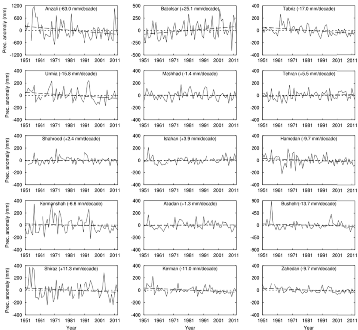
شکل ۸. تغییرات سالانه بی‌هنجاری بارش در ۱۵ ایستگاه همدیدی ایران برای دوره ۱۹۵۱-۲۰۱۳، به‌همراه رگرسیون خطی و مقدار تغییرات در هر دهه.
