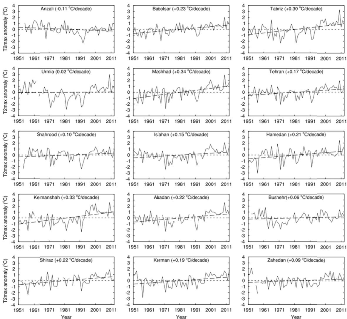
شکل ۵. تغییرات سالانه بی‌هنگاری دمای بیشینه در ۱۵ ایستگاه همدیدی ایران برای دوره ۱۹۵۱-۲۰۱۳، به همراه رگرسیون خطی و مقدار تغییرات در هر دهه.
