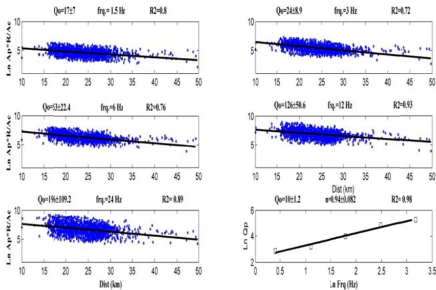
شکل ۵. برآورد ضریب کیفیت امواج تراکمی به روش نرمال‌سازی کدا در منطقه فاریاب در ۵ بازه فرکانسی برای پرتوهای لرزه‌ای امتدادشان عمود بر شکستگی زلزله اصلی است. در هر یک از پنج بازه فرکانسی نسبت Ln دامنه‌ها بر حسب فاصله رسم شده است. در شکل آخر Ln Qp بر حسب Ln Freq رسم شده و مقدار Q0 برای پرتوهایی که عمود بر ساختارهای طی مسیر کرده‌اند، به دست آمده است.
