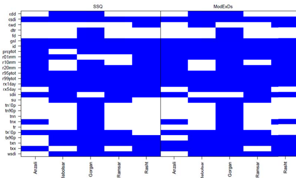
شکل ۳. آزمون مقایسه توزیع شاخص‌های فرین دما و بارش مشاهداتی و شبیه‌سازی شده با استفاده از دو روش SSQ و ModExDs طی دوره اعتبارسنجی (۱۹۹۱-۲۰۱۳).
