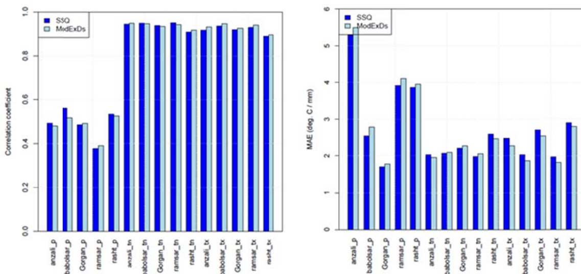
شکل ۶. نمودار همبستگی پیرسون (چپ) و میانگین خطای مطلق (راست) مقادیر مشاهداتی و شبیه‌سازی‌شده ایستگاه‌های مورد بررسی طی دوره اعتبارسنجی (۲۰۱۳-۱۹۹۱).
