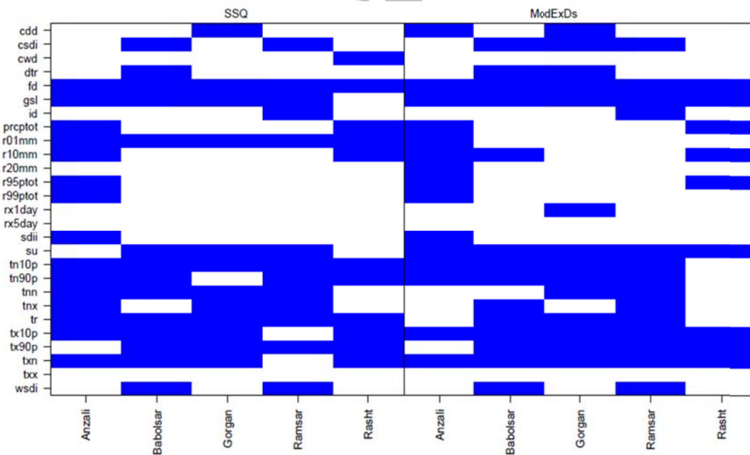
شکل ۲. آزمون مقایسه همبستگی شاخص‌های فرین دما و بارش مشاهداتی و شبه‌سازی شده با استفاده از دو روش SSQ و ModExDs طی دوره اعتبارسنجی
