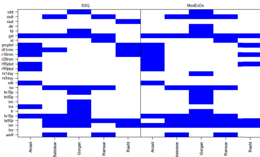
شکل ۴. آزمون ترکیبی ارزیابی روش‌های SSQ و ModExDs بر اساس شاخص‌های فرین دما و بارش طی دوره اعتبارسنجی (۱۹۹۱-۲۰۱۳).
