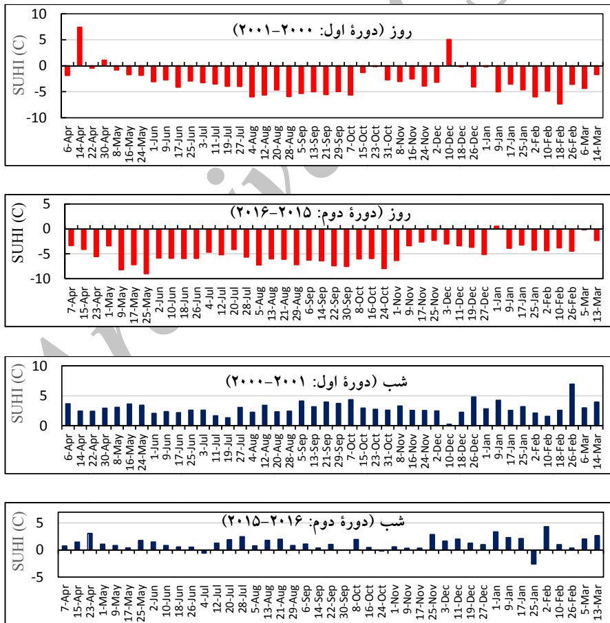
شکل ۵. مقدار شاخص جزیره گرمایی سطحی شهری (SUHI) کرمانشاه در شب و روز با تصاویر مادیس (برای یاخته‌های معرف) در دو دوره یک‌ساله اول
