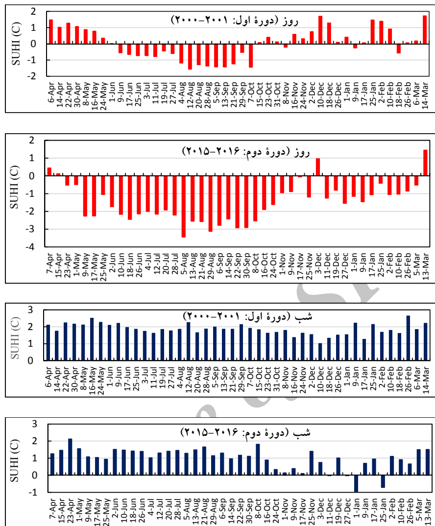
شکل ۳. مقدار شاخص جزیره گرمایی سطحی شهری (SUHI) کرمانشاه در شب و روز با تصاویر مادیس (میانگین تمام یاخته‌ها) در دو دوره یک‌ساله اول (۲۰۰۱-۲۰۰۰) و دوم (۲۰۱۶-۲۰۱۵).
