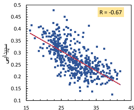
دمای سطح زمین (سانتیگراد)
