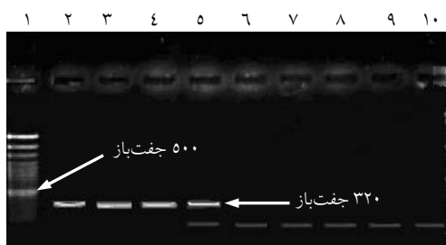
شکل ۳ تعیین حساسیت بر حسب میزان غلظت DNA ژنومی باکتری نیسریا مننژیتیدیس که حساسیت 4500 \text{ CFU/ml} برای نیسریا مننژیتیدیس مشخص شد. ستون ۱: این ستون مربوط به نشانگر ۱۰۰ جفت‌باز است، ستون‌های ۲ تا ۱۰: این ستون‌ها مربوط به رقت‌های 10^{-1} تا 10^{-9} DNA ژنومی این باکتری است.
