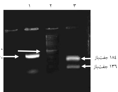
شکل ۲ برش آنزیمی محصول PCR (نیسریا مننژیتیدیس). ستون ۱: محصول PCR. ستون ۲: Ladder ۱۰۰ جفت‌باز، ستون ۳: قطعات حاصل از برش آنزیمی opa
