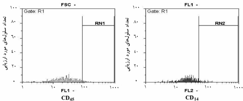
شکل ۵ ارزیابی سلول‌های حاصل از هم‌کشتی U266 و HSC از نظر نشانگرهای (RN1) CD 45 و (RN2) CD 14
