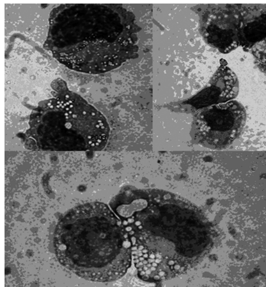
شکل ۲ رنگ‌آمیزی TRAP سلول‌های حاصل از هم‌کشتی U266 و U937؛ وجود واکوئول‌های متعدد در سیتوپلاسم سلول‌ها و نقاط قرمز که نتیجه مثبت بودن رنگ‌آمیزی TRAP در آن‌ها است. (بزرگنمایی: ۱۰۰ ×)
