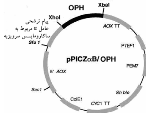
شکل ۱ نمای شماتیکی از ناقل pPICZαB حاوی ژن OPH (ناقل نو ترکیب)
