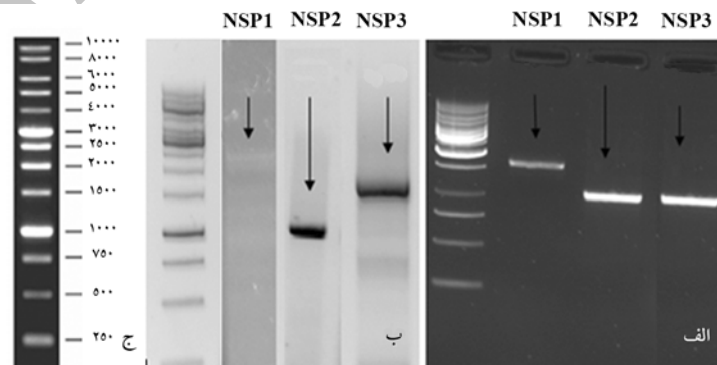
شکل ۳ (الف) الکتروفورز حاصل از تکثیر قطعات استاندارد، (ب) الکتروفورز حاصل از قطعات بازآرایی شده، (ج) نشانگر ۱ کیلو بایز #SM0311
