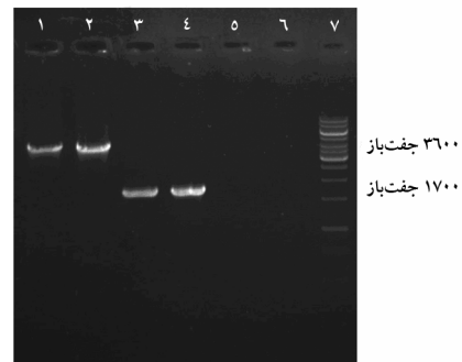
شکل ۳ الکتروفورز ژل آگارز برای محصولات PCR روی DNA ژنومی سلول‌های پایدار شده با ناقل‌های pMTPA، pTPA و سلول‌های CHO ترانسفکت نشده (کنترل)؛ ستون‌های ۱ و ۲ سلول‌های پایدار شده با ناقل pMTPA، ستون‌های ۳ و ۴ سلول‌های پایدار شده با ناقل pTPA، ستون‌های ۵ و ۶ سلول‌های CHO کنترل و ستون ۷ نشانگر DNA
