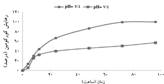
شکل ۴ نمایه رهایش کورکومین از نانو ذره پلی یورتان در دو \text{pH} متفاوت 7/4 (بافر فسفات) و 5/4 (بافر سیترات)
