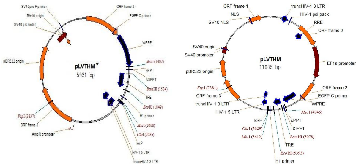
شکل ۲ نقشه حامل‌های pLVTHM* و pLVTHM ترسیم شده با نرم‌افزار Vector NTI؛ اندازه حامل pLVTHM از ۱۱ کیلوباز به ۶ کیلو باز در pLVTHM* کاهش یافت. shRNA در بین دو جایگاه برشی MluI و ClaI کلون شد.
