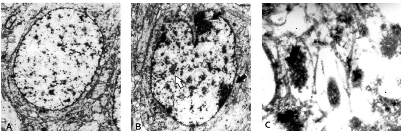
شکل ۱. میکروسکوپ الکترونی از هیپوکامپ (A) گروه کنترل (B) گروه سرب (C) گروه سرب + ویتامین ث. در گروه B علایم آپتوز از جمله تراکم کروماتین (پیکان سفید) مهاجرت هستک به محیط (پیکان سیاه) و چین خوردگی های غشای هسته مشاهده می شود. (بزرگنمایی: A, B: ۱۰۰۰۰×-A, B: ۳۰۰۰۰×) (C)
