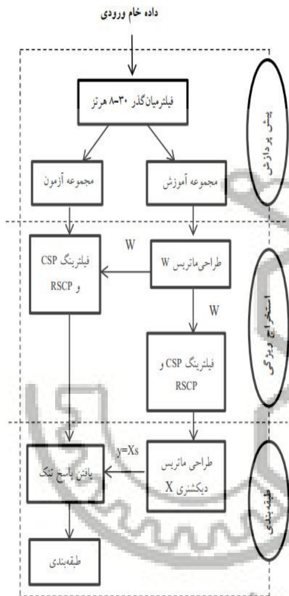
شکل (۷) - روندنمای روال کلی مراحل انجام آزمایش‌ها
