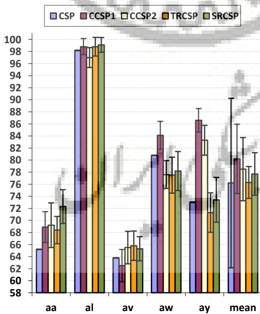
شکل (۹) - میزان میانگین و انحراف معیار درصد صحت طبقه‌بندی برای افراد مختلف با الگوریتم OMP
