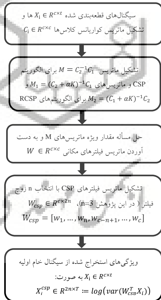
شکل (۵) - روندنمای روال استخراج ویژگی به روش‌های CSP و RCSP
