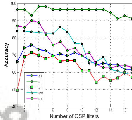
شکل (۴) - میزان درصد صحت تشخیص به‌ازای زوج فیلترهای مختلف برای الگوریتم CCSP1
