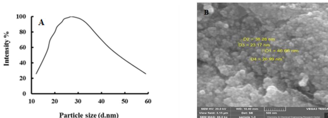
شکل ۲-۲: نتایج حاصل از اندازه گیری اندازه نانوذرات نقره به کمک تکنیک (A) DLS و (B) SEM
