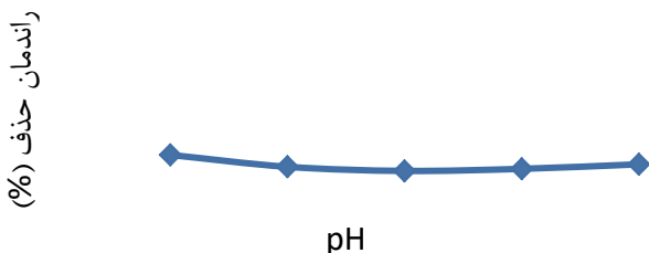
شکل ۳. تعیین اثر pH بر بازده حذف کروم شش ظرفیتی در دوز جاذب ۸ g/L، غلظت اولیه کروم شش ظرفیتی ۵۰ میلی گرم بر لیتر، دور اختلاط ۲۵۰ دور بر دقیقه و زمان واکنش ۱۲۰ دقیقه
