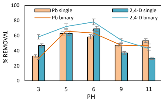
شکل ۴. الف. تأثیر pH بر جذب سرب و 2,4-D در سیستم جذب مجزا و همزمان توسط نانوذرات مغناطیسی Fe_3O_4@SiO_2-NH_2-SH (غلظت اولیه ۲۵ mg/L و دوز جاذب ۰/۴ g/L در سیستم مجزا و ۰/۸ g/L در سیستم همزمان، دمای ۲۵ °C)
