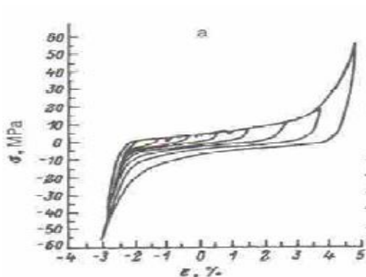
شکل ۷- نمودار تنش - کرنش (اقتباس از مرجع [۷]).
