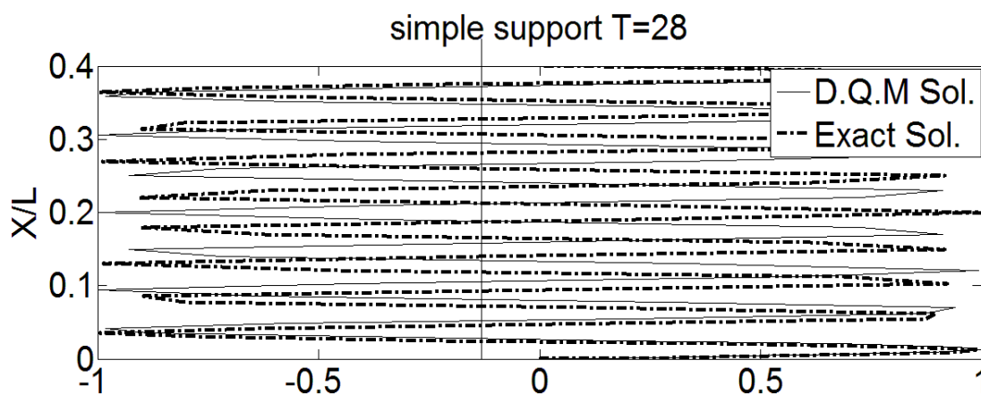
شکل ۹- نمودار مود کمانش استوانه جدار نازک در حالت تکیه گاه ساده بدست آمده از حل دقیق و DQM در دمای ۲۸ درجه.
