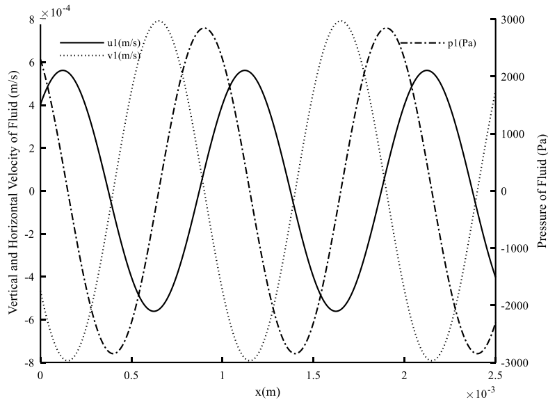
شکل ۴- پروفیل فشار و مؤلفه‌های سرعت در جهت مماس بر سطح در فاصله ۰/۲ میکرون از کف
